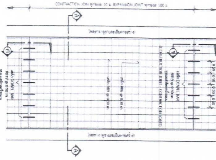
แบบขยาย CONSTRUCTION JOINT และ CONTRACTION JOINT ทุกระยะ 10 เมตร
